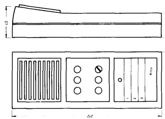
Maßskizze 9263...
